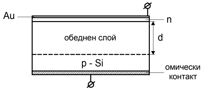
Фиг.58. Схема на повърхностно-бариерен Si детектор.
