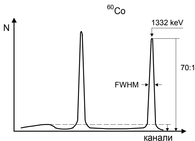
Фиг.57. Към параметрите на HpGe детектора в лабораторията по Експериментална ядрена физика.
