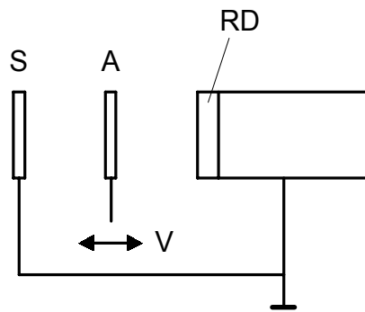
Фиг.139. Схема на постановка за снемане на спектри на проби с резонансен детектор: S – източник, A – абсорбер, RD – резонансен детектор, V – скорост (вibrator).
