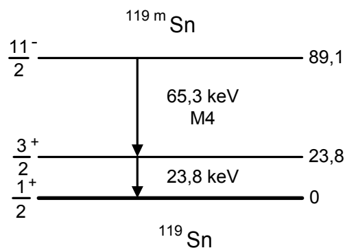
Фиг.135. Схема на разпад на изомера ^{119m}\text{Sn} .
