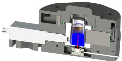
ФИГУРА 7.1: Разрез на C-TDCR детекторната система. Червената линия показва лъча на външния източник на \gamma -лъчи. Фигурата беше предоставена за използване в дисертацията от Беноа Сабо (LNE-LNHB).
