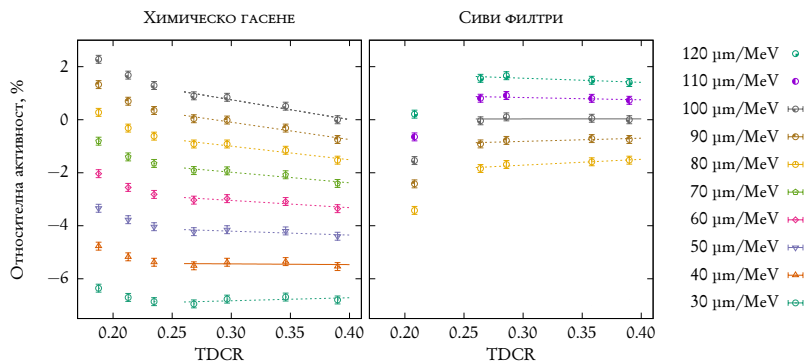
ФИГУРА 6.5: Относителна активност като функция на TDCR параметъра при намаляване на ефективност с химическо гасене и сиви филтри. Линейния фит с наклон най-близък до нулата е показан с плътна линия.
