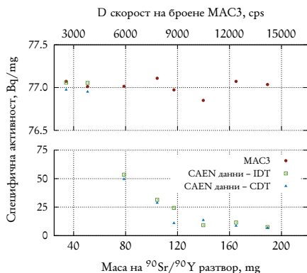
ФИГУРА 2.3: Специфична активност на източник ^{90}\text{Sr}/^{90}\text{Y} с постановка №1.
